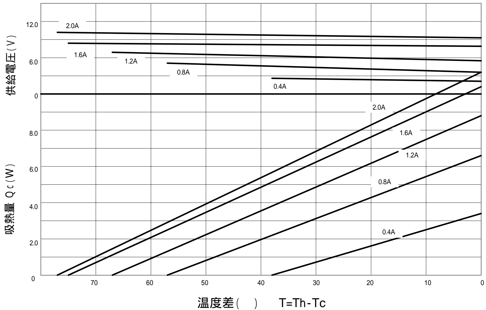
FPH1 - 7102M 特性図 (Th=50 )
