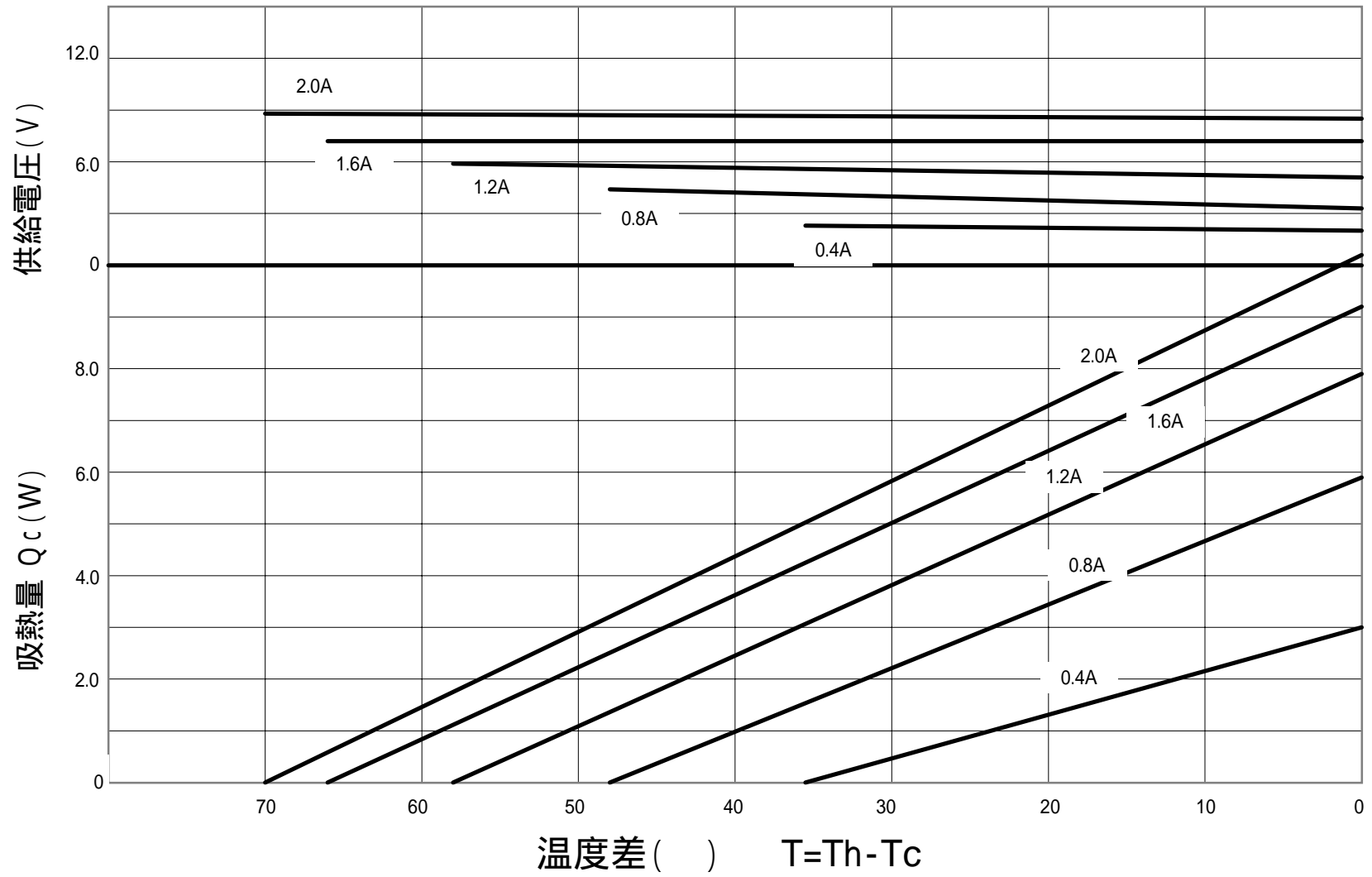
FPH1 - 7102M 特性図(Th=27 )
